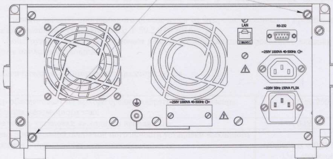
Рисунок 2 - Схема пломбирования прибора
